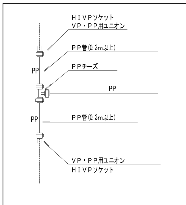
キ 「VP」 「HIVP」 口径40mm以下の切取り工事
